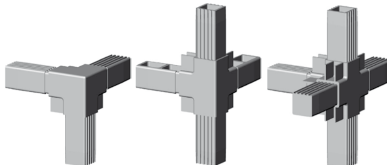
Steckverbinderserie für Quadratrohr 25x25 mm mit Stegen am Würfel Plug-in connector range 25x25 mm with bridges at the cube Gamme de raccords multiples 25x25 mm avec des passerelles au cube
